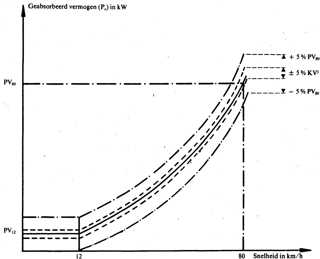
Diagram van het door de rollenbank geabsorbeerde vermogen
