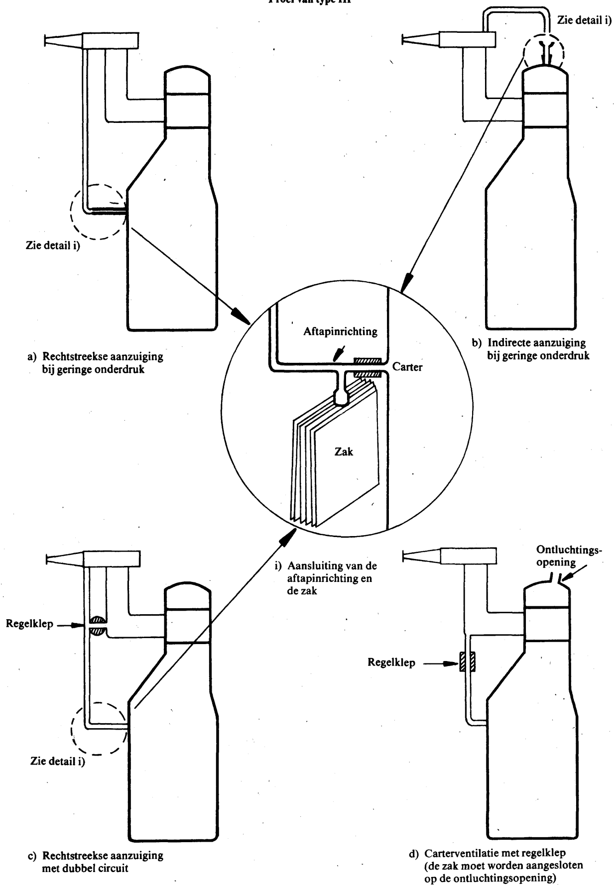
Figuur V. 5 Proef van type III
