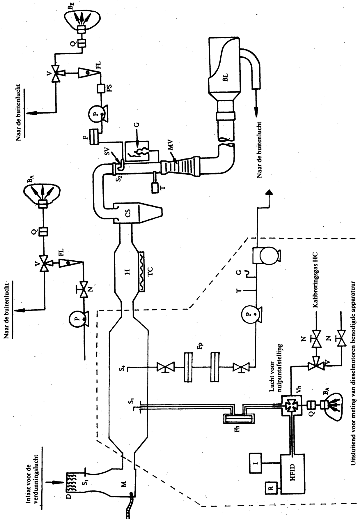
Figuur III.5.3.2 Schema van een monsterningssysteem met constant volume met gebruik van een venturibus met kritische stroming (CFV-CVS)
